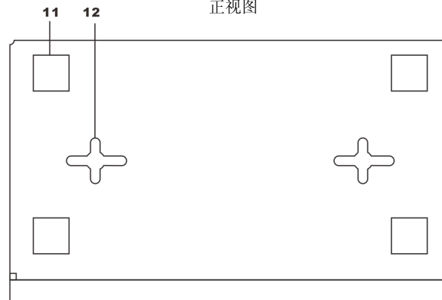
仰视图
