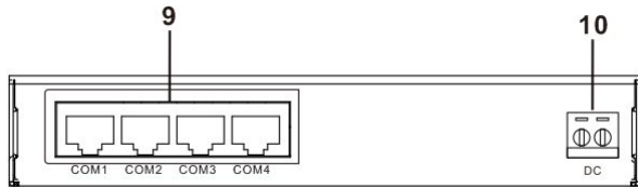
后视图
