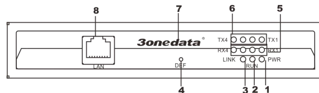
正视图
