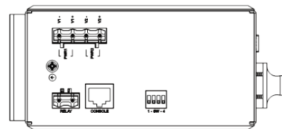
俯视图
