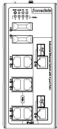
主视图：IPS7110-6T2F2GC-4POE
