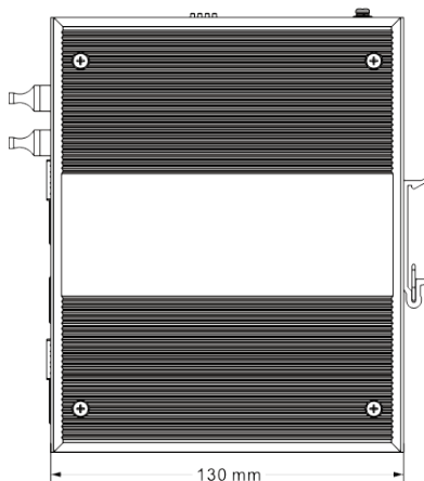
侧视图
