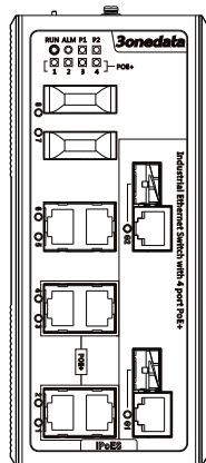
主视图: IPS3110-6T2F2GC-4POE
