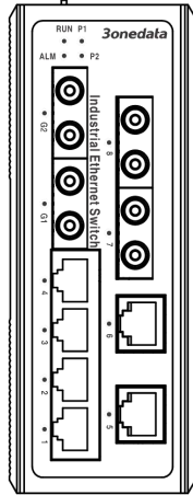
IES2010-2GF-2F 前视图
