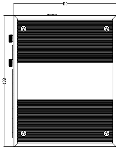
侧视图
