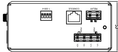
俯视图
